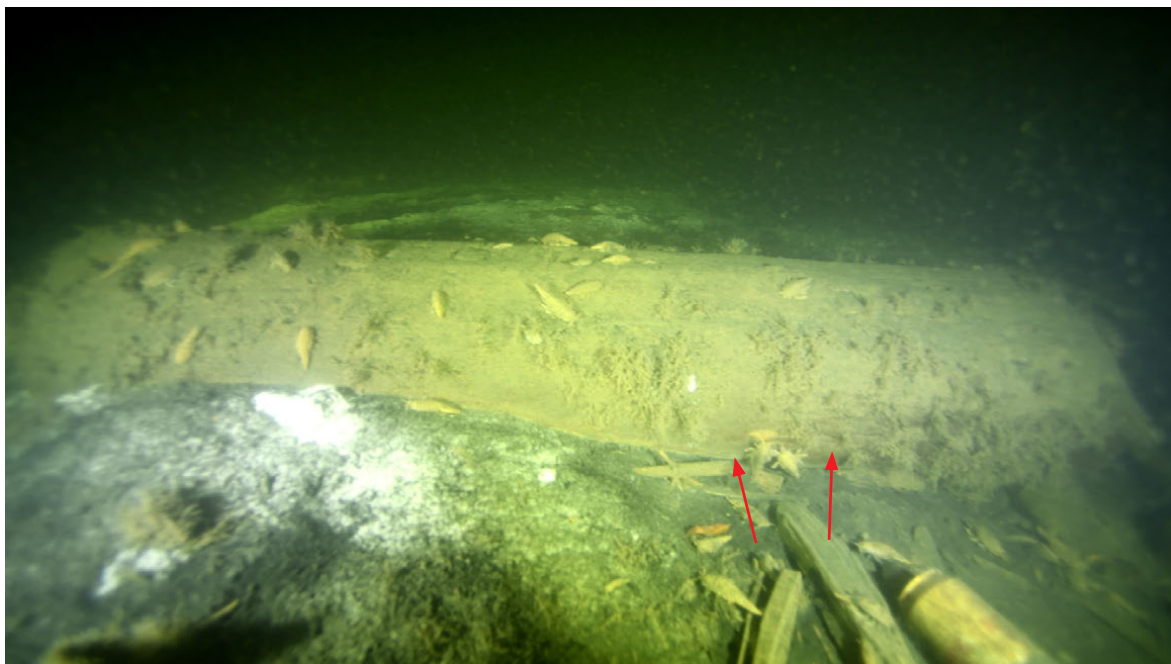
FIGUR 55. Timret påminner mycket om Id "Timmer hett". Det lite mer beväxning men två hål för trädymlingar syntes (se röda pilar). Foto: Jim Hansson, Vrak – Museum of Wrecks/SMTM. Digitalt museum: VK.V 0258.
