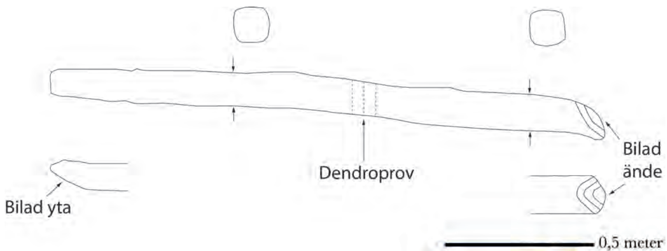
Figur 293. Timmer 50 Ritning: Andreas Olsson, Statens maritima museer
