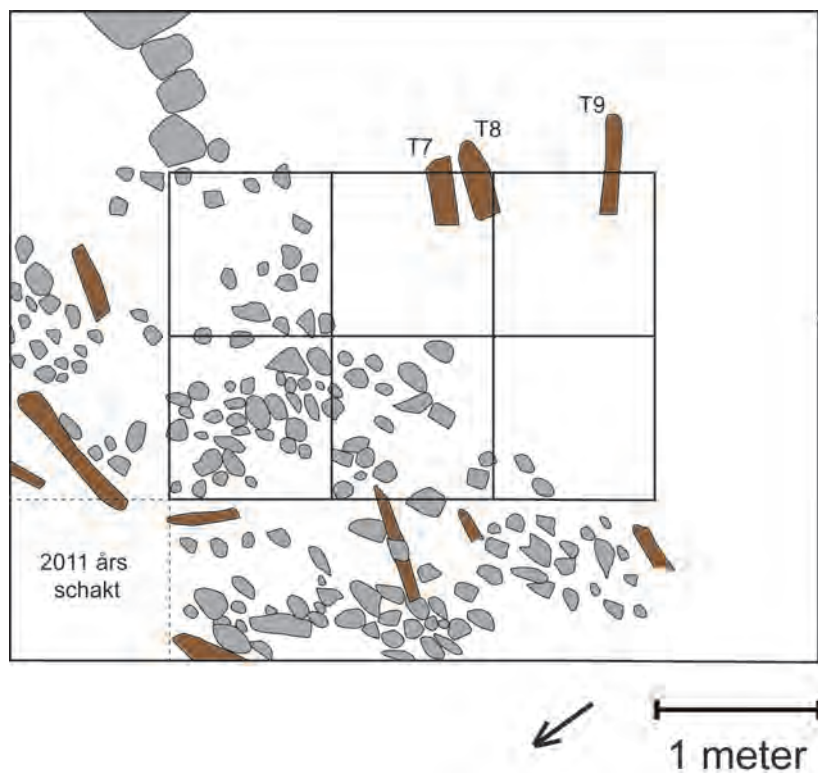
Figur 258. Plan över det underliggande stenlagret. Endast stenarna inom schaktbegräns-ningen togs helt och hållet bort. Ritning: Andreas Olsson, Statens maritima museer.
