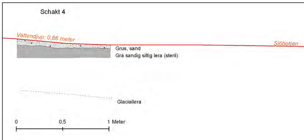
Figur 20. Profil över provgrop 4 ritad från norr. Ritning: Jens Lindström, Statens Maritima Museer.
