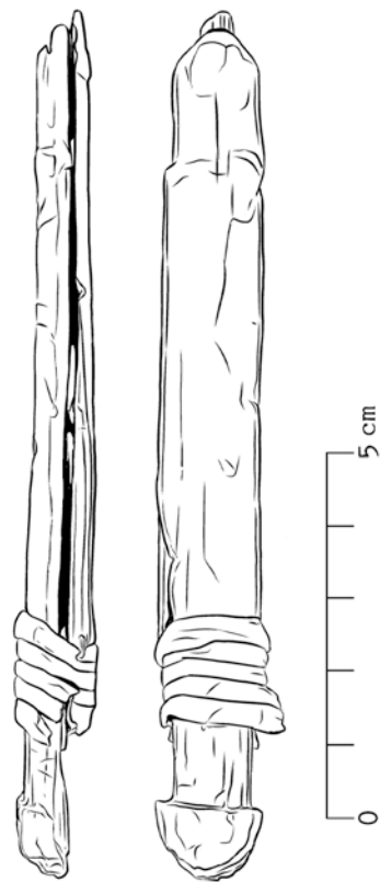
Figur 205. Fyndnummer 140, laggbandsavslut som liknar ett svärd? Illustration: Marit Furn, Statens maritima museer.
