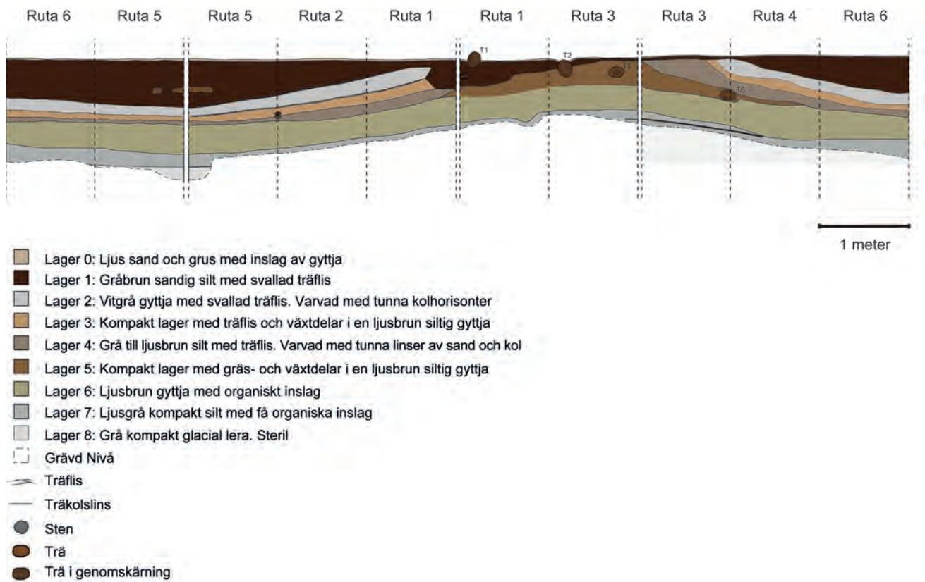
Figur 164. Samtliga fyra profilritningar i schaktet lagda efter varandra. Ritning: Andreas Olsson, SMM.
