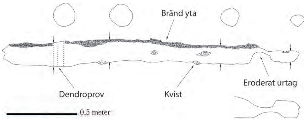
Figur 294. Timmer 57, Ritning: Andreas Olsson, Statens maritima museer.
