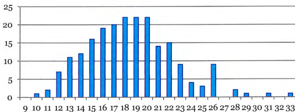
Figur 340. Antal fartygsrelaterade tränaglar, av olika diametrar, från Hedeby. Den horisontella axeln representerar diameter i millimeter och den vertikala representerar antal tränaglar. Tabellen är baserad på information från Crumlin-Pedersen 1997:122, tabell 5.3.
