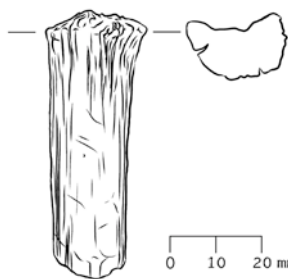
Figur 207. Fyndnummer 31, halverad tränagel med brutet skaft. Illustration: Marit Furn, Statens maritima museer.
