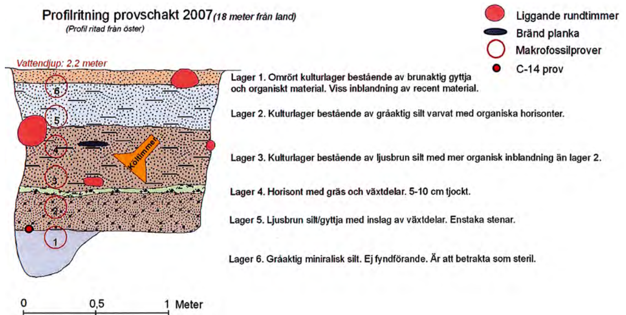
Figur 15. Profilritning över provgroppen från 2007. Profilen visar den västra sidan. Ritning: Jens Lindström
