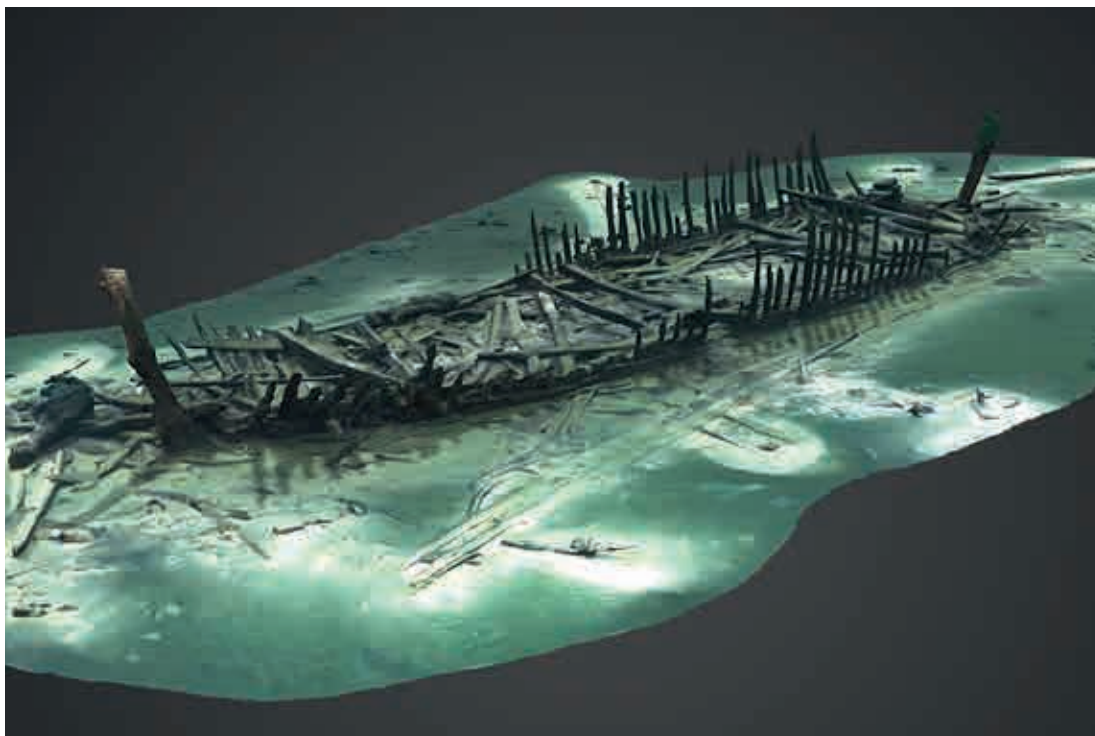
3D-modell av Resande Mans vrakplats. Spanten reser sig fortfarande högt på vraket.
